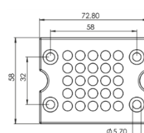
KEL-DPZ-B 25
