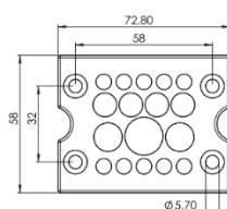
KEL-DPZ-B 17
