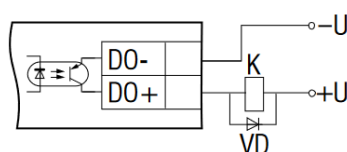
NPN-Transistorausgang / NPN-transistor output
