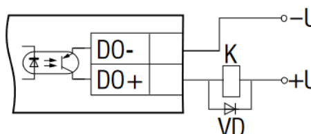
NPN-Transistorausgang / NPN-transistor output
