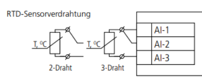
RTD-Sensorverdrahtung / RTD - sensor wiring
