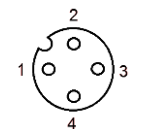
4 POLIG / 4-pole
