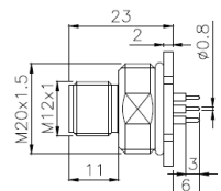
Version mit Lötkontakten / version with soldering contacts
