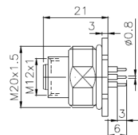
Version mit Lötkontakten / version with soldering contacts
