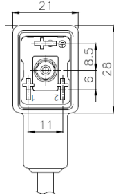
DIN Form B-Industrie
