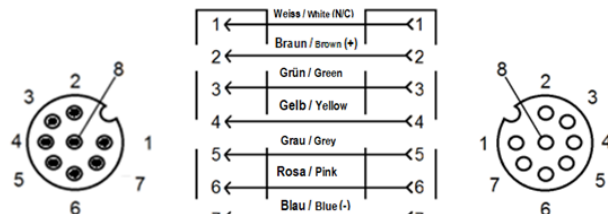
8 POLIG / 8-pole
