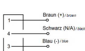
3 POLIG / 3-pole
