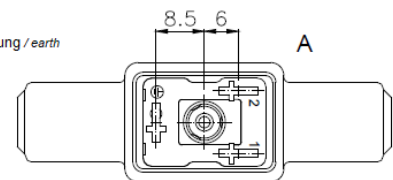
H6 Erdung / earth
