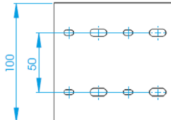
VK 100mm Breite/Width/Largeur
