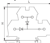
Nq4-Diode V4
