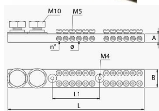
KL11-2x6 - KL11-2x24
