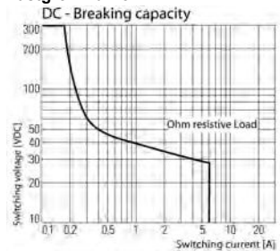
Lastgrenzkurve
