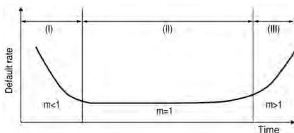
Badewannenkurve
