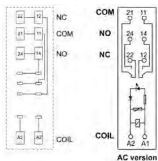
Relaissockel für Industrierelais
