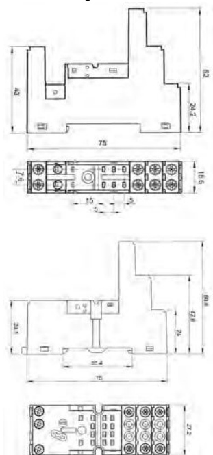
Anschlussbild
