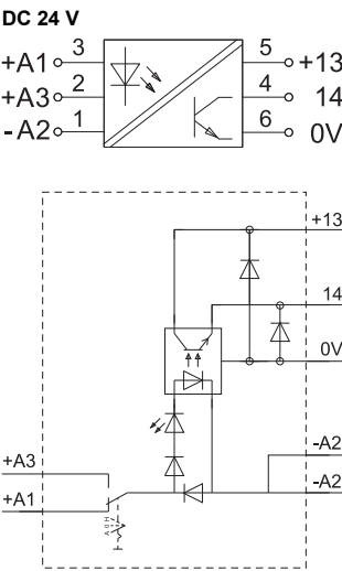
Anschlussbild
