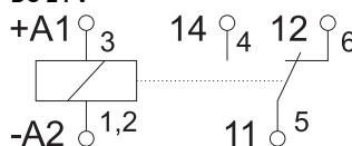
Anschlussbild
