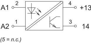
Anschlussbild
