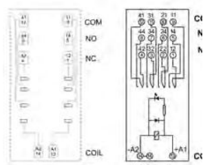
Relaissockel für Industrierelais
